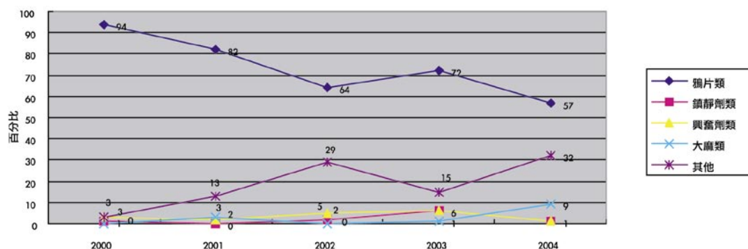
圖5. 吸毒種類一直以海洛英為主，過去約佔90%，但近年已有下降之趨勢，由2000年之95%下降至2004年最低之75%。其他類之毒品比例則不斷上升。
